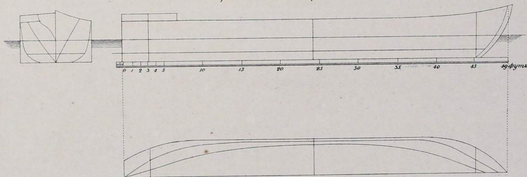
Чертежъ XIII къ фиг. 18 и 20.
