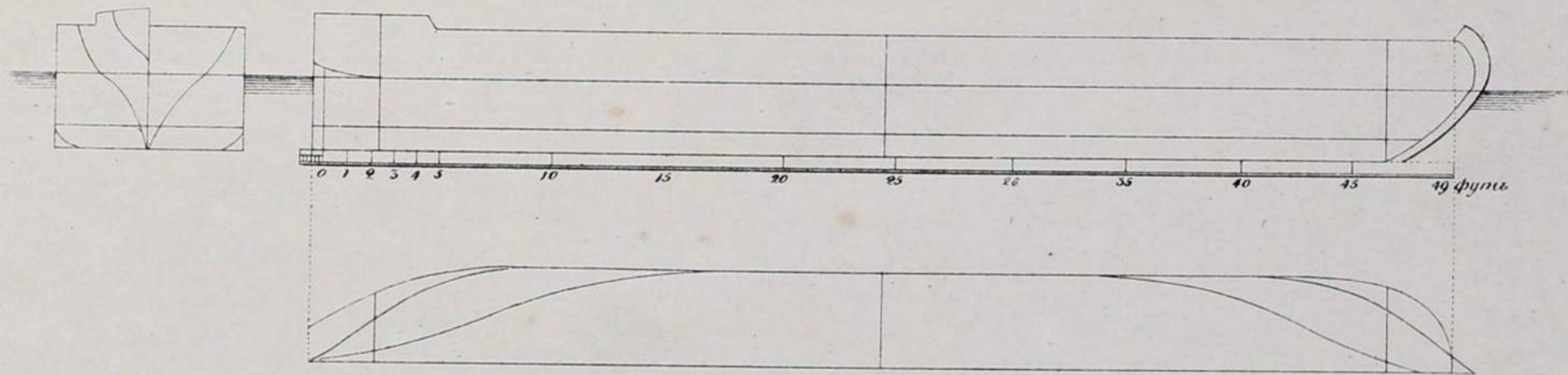
Чертежъ VIII къ фиг. 21.
