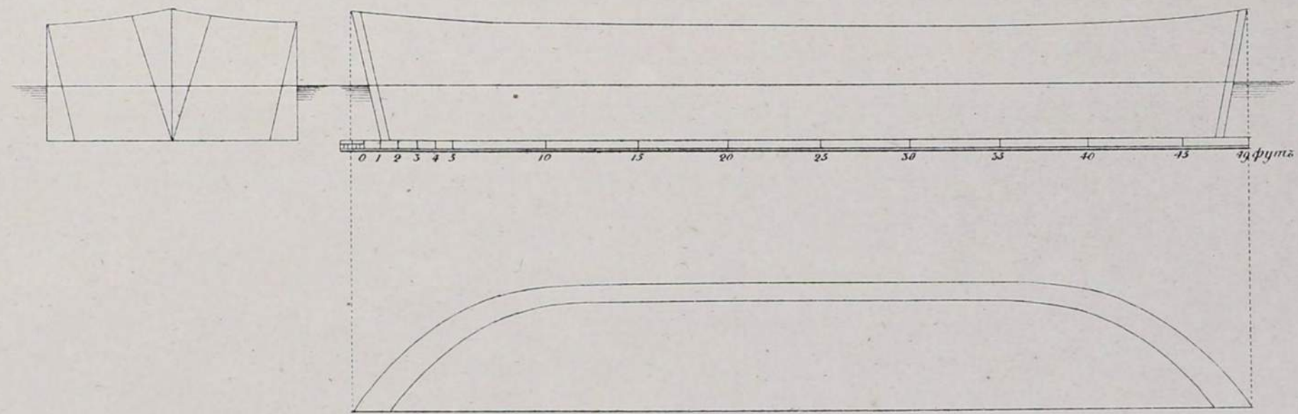
Чертежъ XII къ фиг. 19, и 64.
