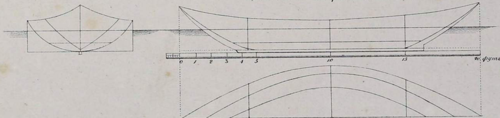
Чертежъ X къ фиг. 28. и 59.
