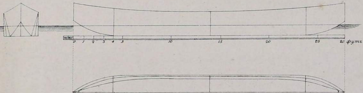
Чертежъ XIX къ фиг. 47 и 48.
