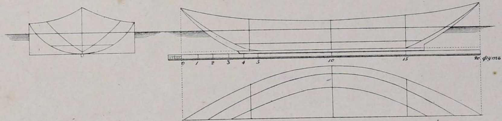
Чертежъ X къ фиг. 56, 57, и 58.
