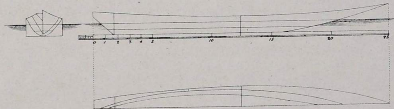
Чертежъ XXI къ фиг. 62 и 63.
