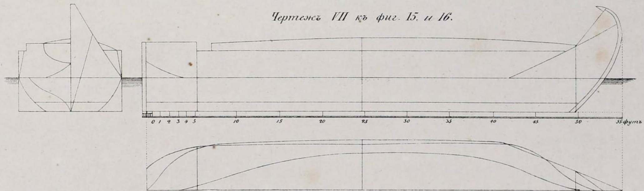
КАЮКЪ.
