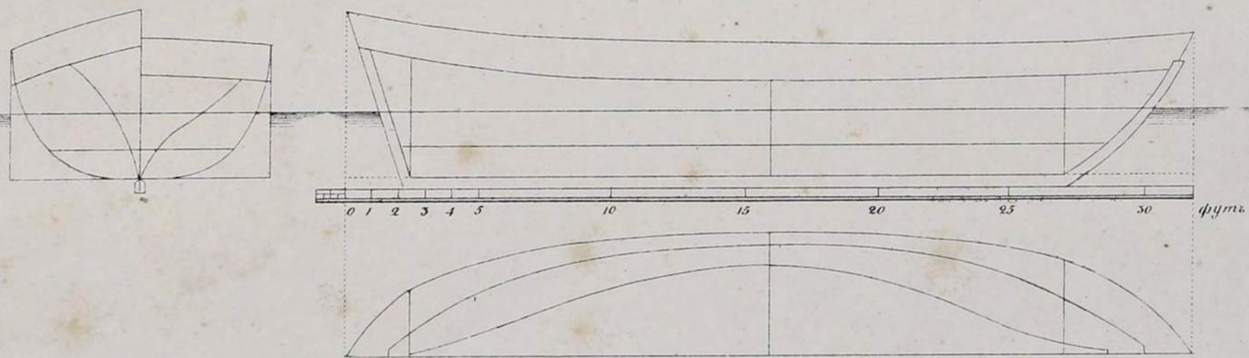
Чертежъ II къ фиг. 4.
