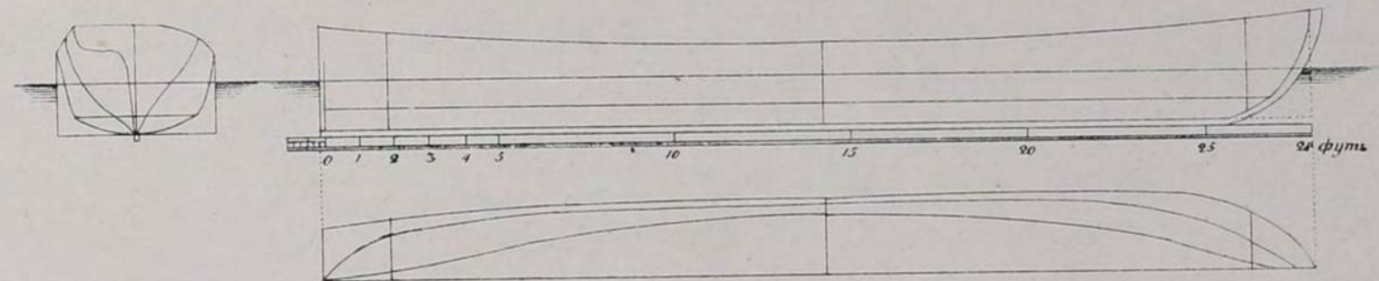
Чертежъ XVIII къ фиг. 46.
