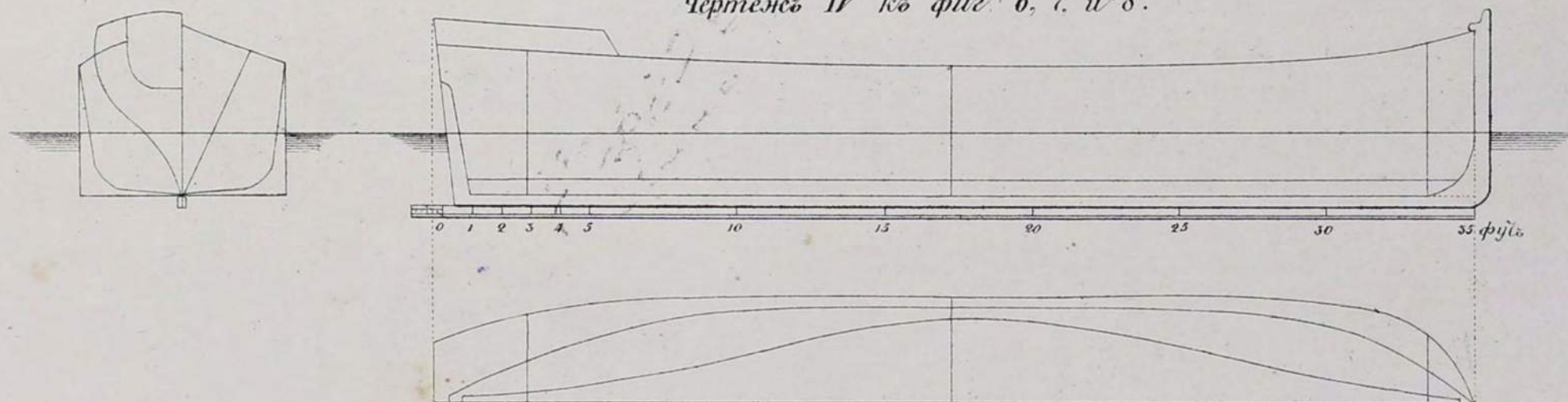
Чертежъ IV къ фиг. 6, 7, и 8.
