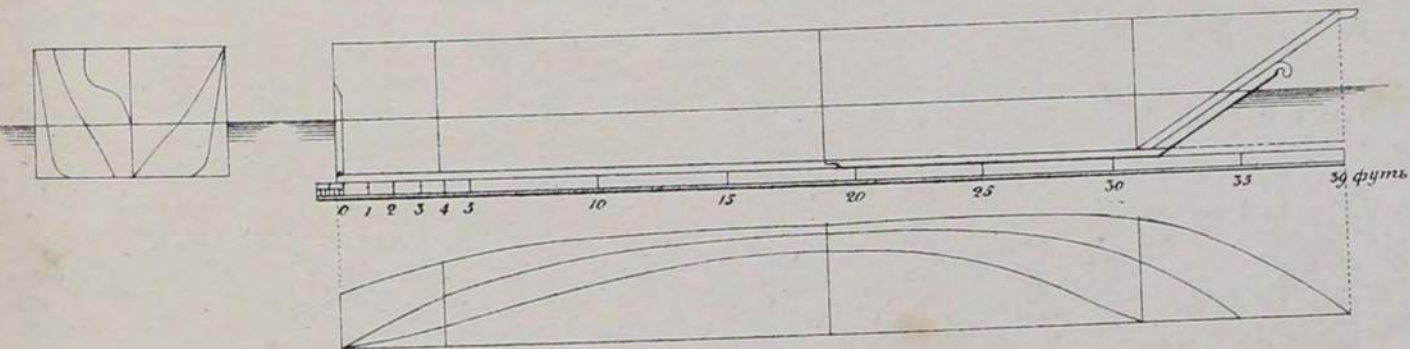
Чертежъ XVII къ фиг. 53.
